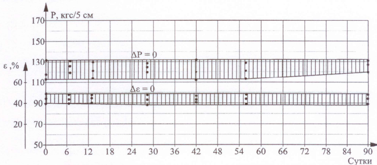
Рис. 3. Изменение прочности (1) и относительного удлинения (2) образцов материала "Техноэластмост Б" при воздействии насыщенного раствора NaCl
